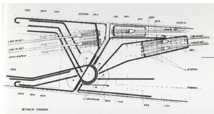
Dettaglio Viadotto Magliana
